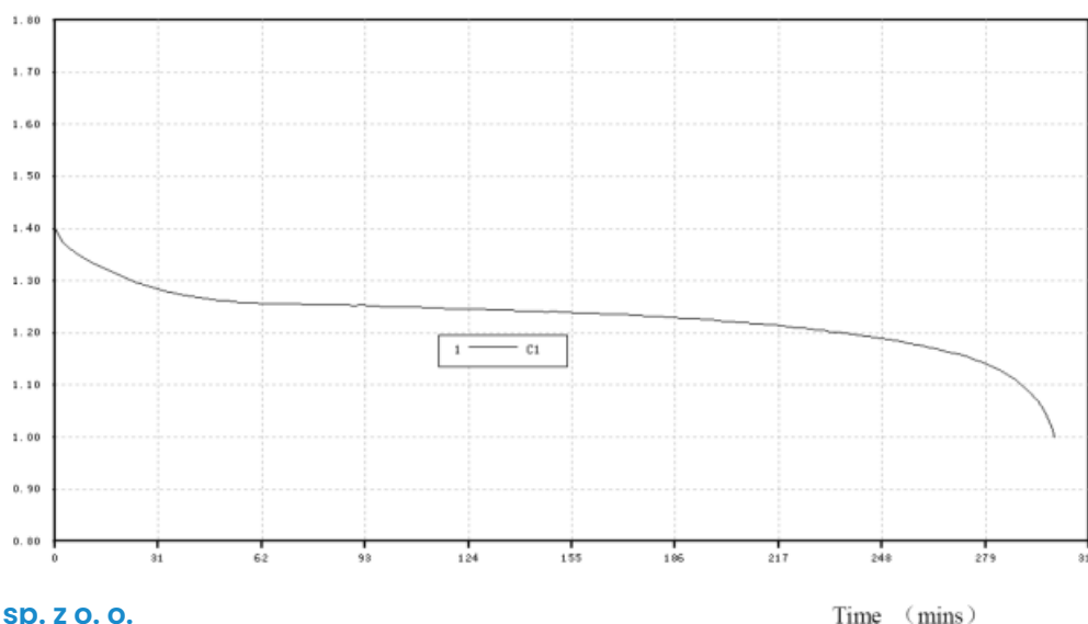
Charakterystyka rozładowania (load 0.2C - 1000 mA):
